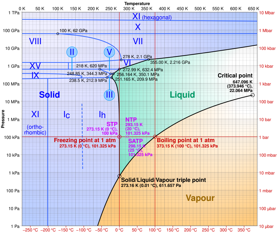
图 12: 冰的相图
